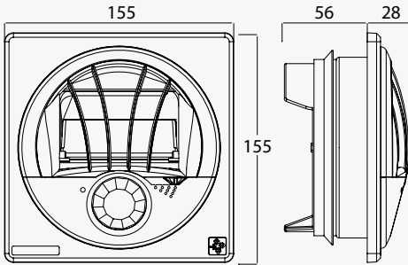
Размеры, мм
