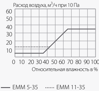
Аэродинамические характеристики
