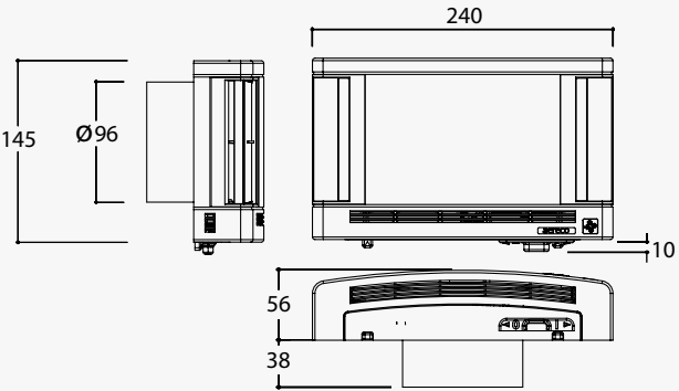
Размеры, мм
