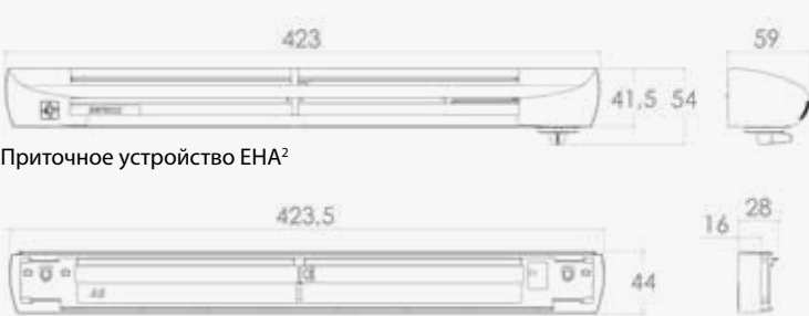
Акустическая проставка E-EHA²
